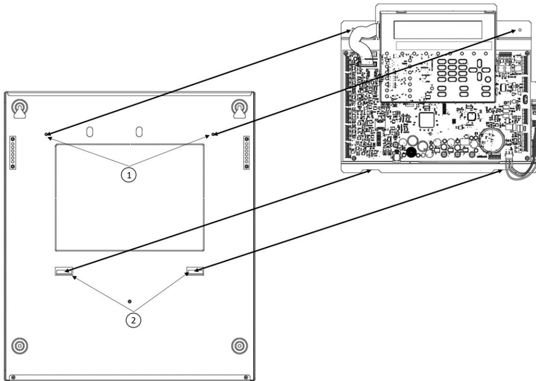
Figura 2: Detalles de montaje del chasis
