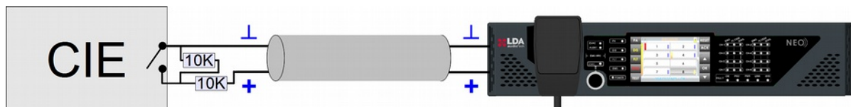
Ilustración 9: Conexión a ECI Supervisada
